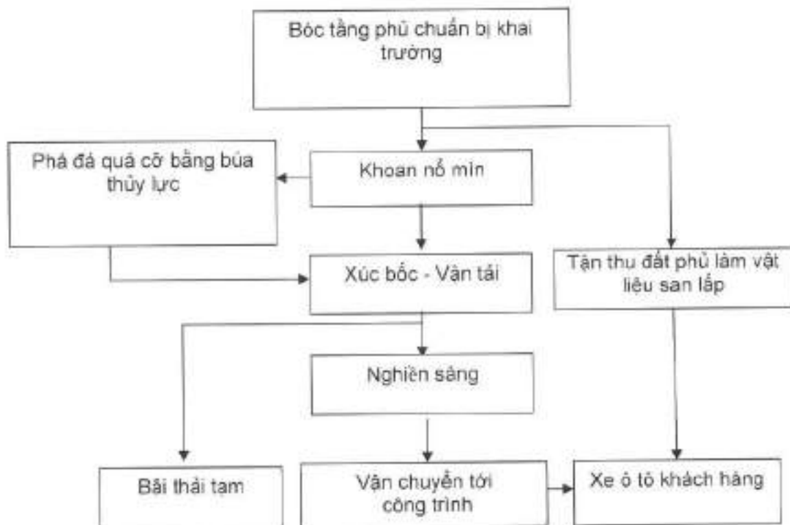
Hình 5. Mô tả sơ đồ công nghệ
